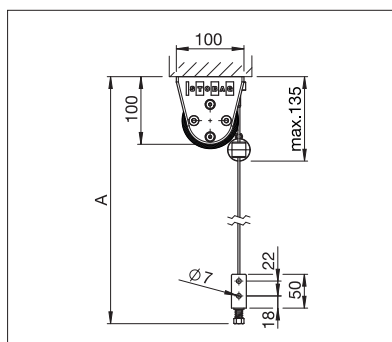
S4110 Montaggio a soffitto con guida
